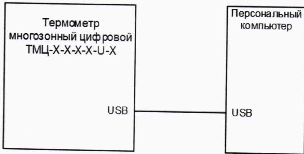
Рисунок А.3 – Схема соединений для проверки абсолютной погрешности измерений температуры и передачи измеренных значений по интерфейсу для модификации ТМЦ-X-X-X-X-U-X
